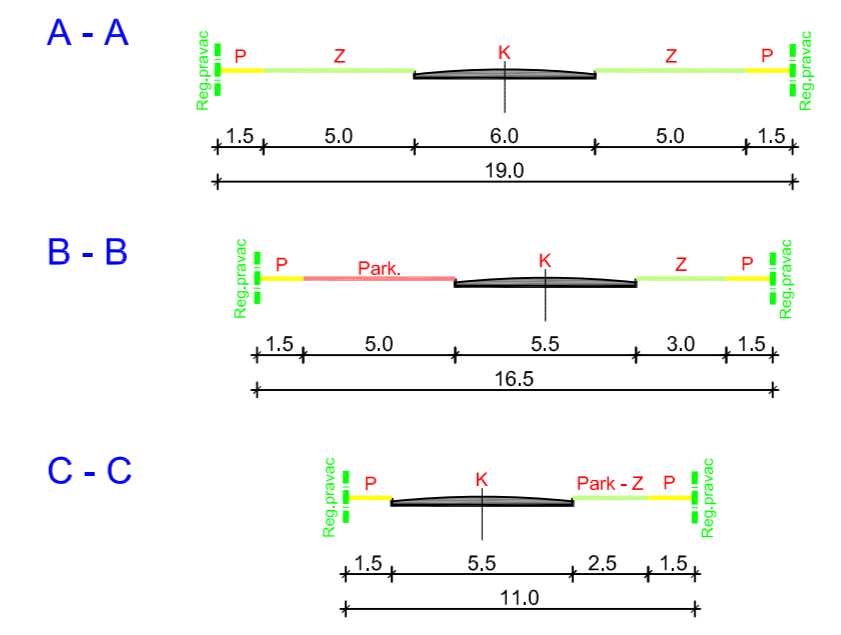
KARAKTERISTIČNI PROFILI PROMETNICA MJ 1:250
