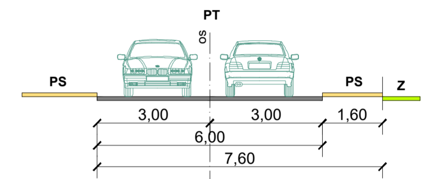
Profil ulice A-A
