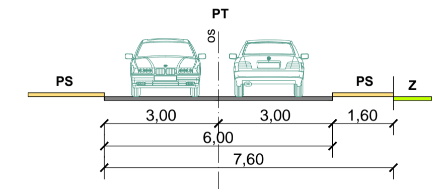
Profil ulice A-A
