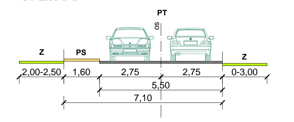
Profil ulice B-B
