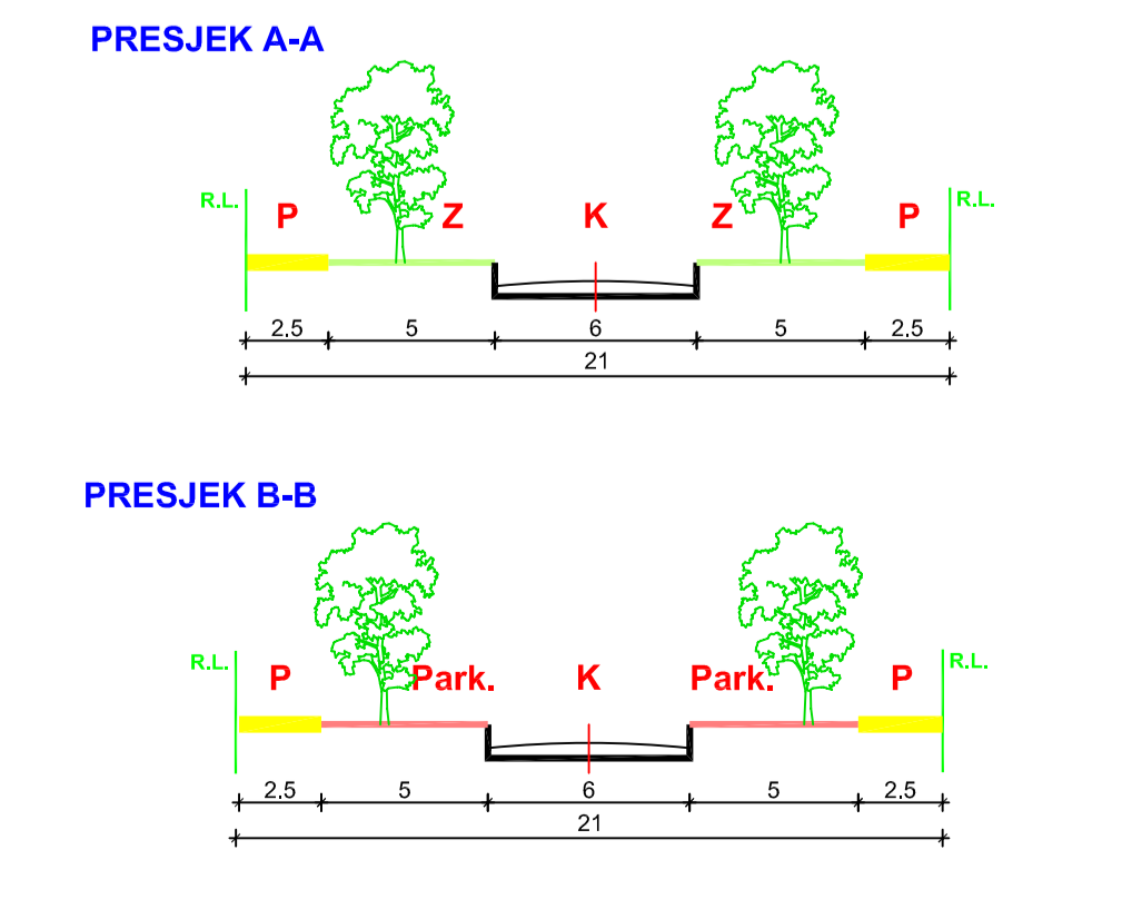
KARAKTERISTIČNI POPREČNI PRESJEK MJ 1:250
