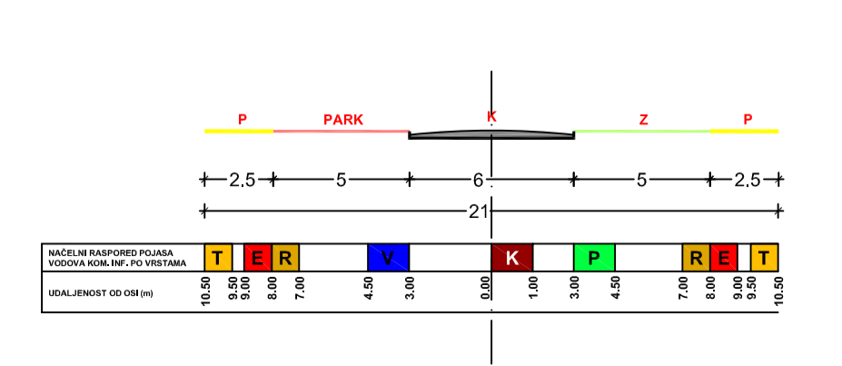
KARAKTERISTIČNI POPREČNI PRESJEK S NAČELNIM RASPOREDOM KOMUNALNE INFRASTRUKTURE MJ 1:250
