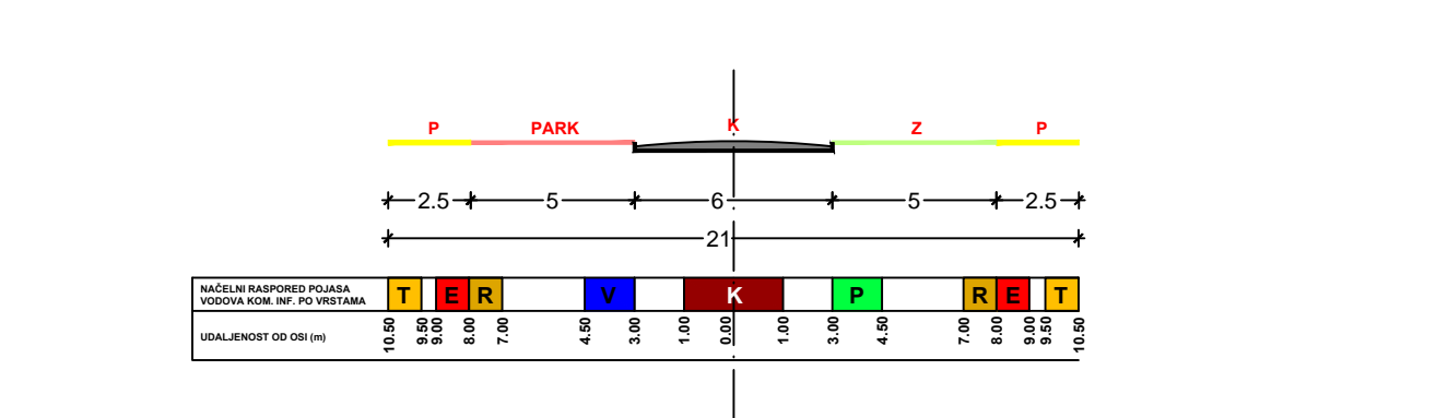
KARAKTERISTIČNI POPREČNI PRESJEK S NAČELNIM RASPOREDOM KOMUNALNE INFRASTRUKTURE MJ 1:250
