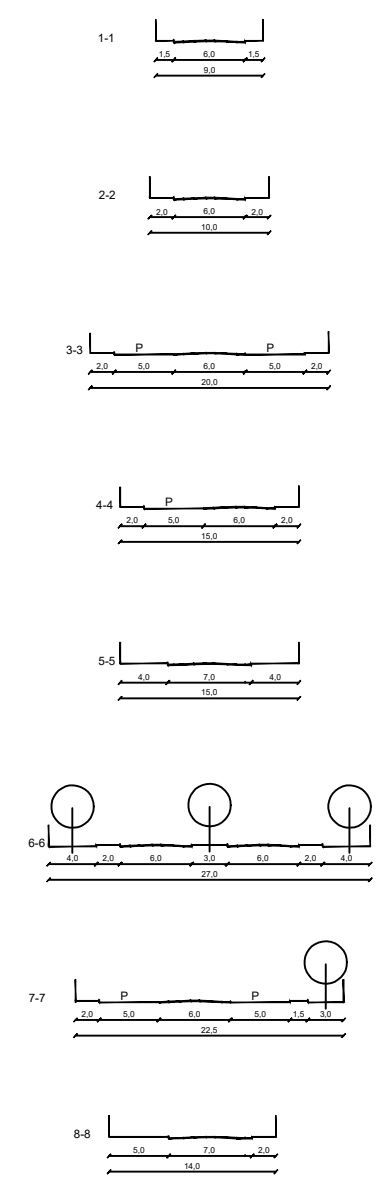
KARAKTERISTIČNI POPREČNI PROFILI PROMETNE MREŽE 1:200
