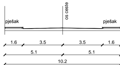
KARAKTERISTIČAN POPREČNI PRESJEK B - B M 1:200
