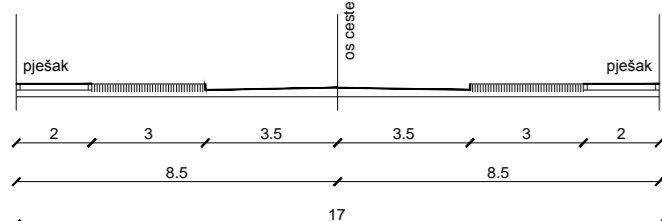
KARAKTERISTIČAN POPREČNI PRESJEK B - B M 1:200
