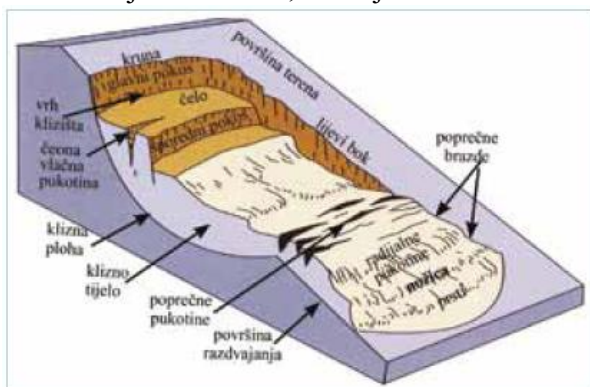
Slike 4: Dijelovi klizišta; Puzanje tla
