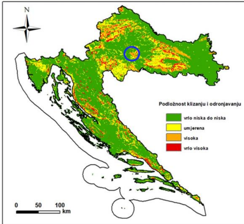
Slika 5: Karta podložnosti na klizanje tla i odrone za Hrvatsku i Grad Kutinu
