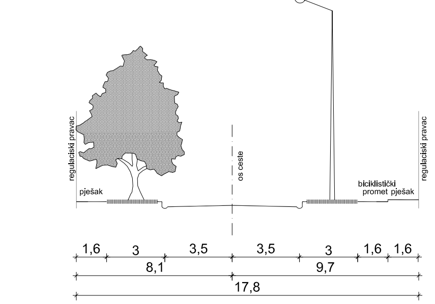
KARAKTERISTIČAN POPREČNI PRESJEK B - B
