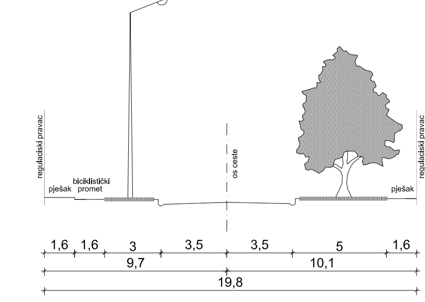
KARAKTERISTIČAN POPREČNI PRESJEK A - A
