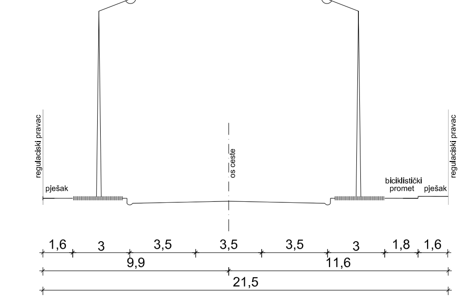
KARAKTERISTIČAN POPREČNI PRESJEK C - C
